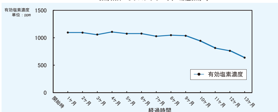
ウィッキル1000 2021年9月9日製造分 経時変化グラフ 保存条件 5ℓ ロンテナー入 常温保存時
