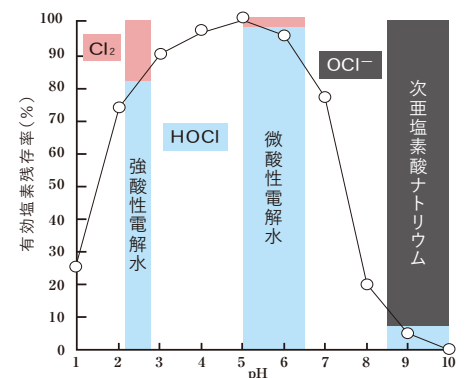
次亜塩素酸(HOCl)の存在比率のpH依存性 酸性で高く、アルカリ性で低い(OCI - に変換)
